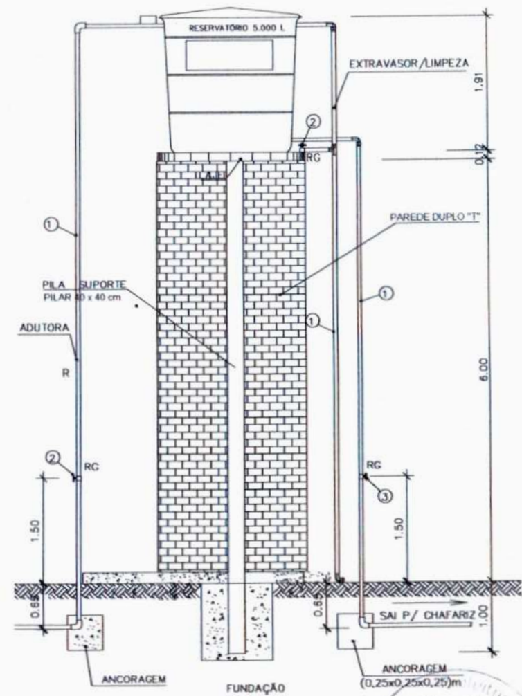
VISTA LATERAL ESC.: 1/50
