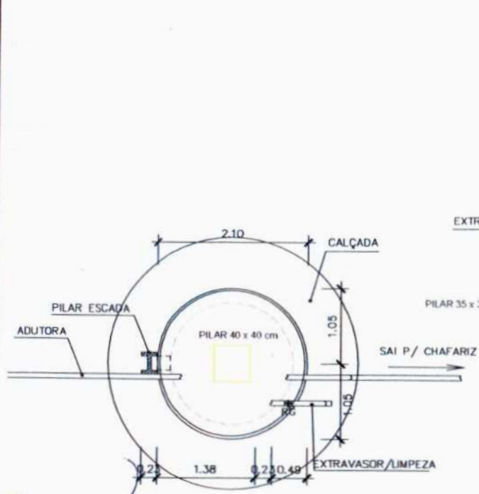
PLANTA BAIXA ESC.: 1/50
