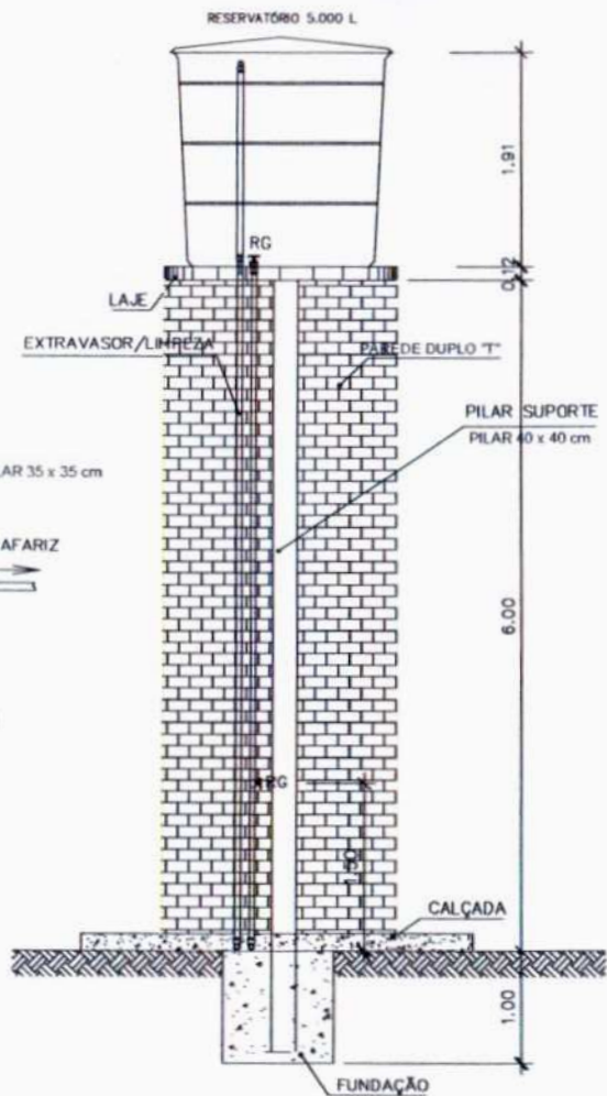
VISTA FRONTAL ESC.: 1/50
